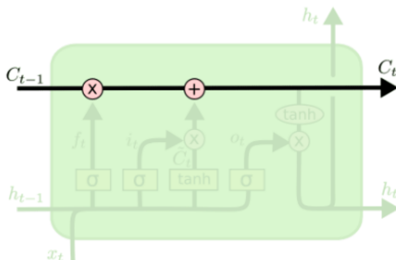
Figura 19. Cell state en la arquitectura LSTM.
